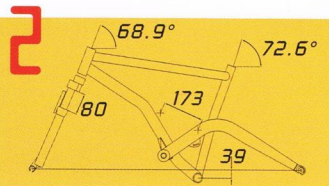
Telaio con "fase negativa". Frame with "negative" phase. Cadre avec "phase négative".
