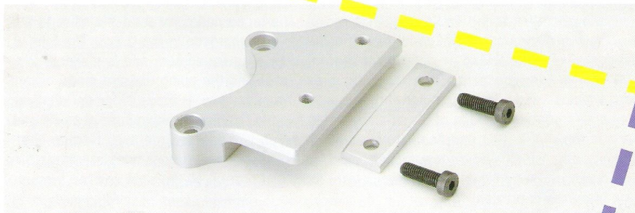
Art. 77.10100 Kit attacco pinza per forcelle MARZOCCHI DH3 Caliper attachment kit for MARZOCCHI DH3 forks
